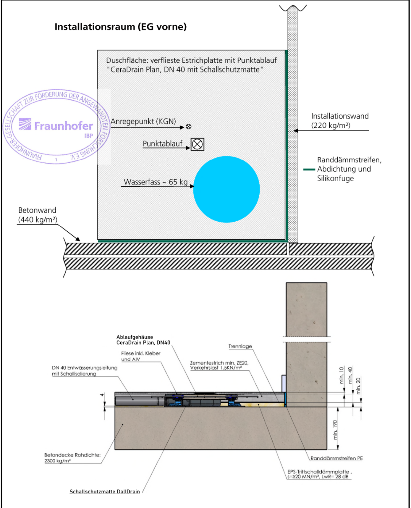
Bild oben: Lage des Prüfaufbaus im Installationsraum (EG vorne).
